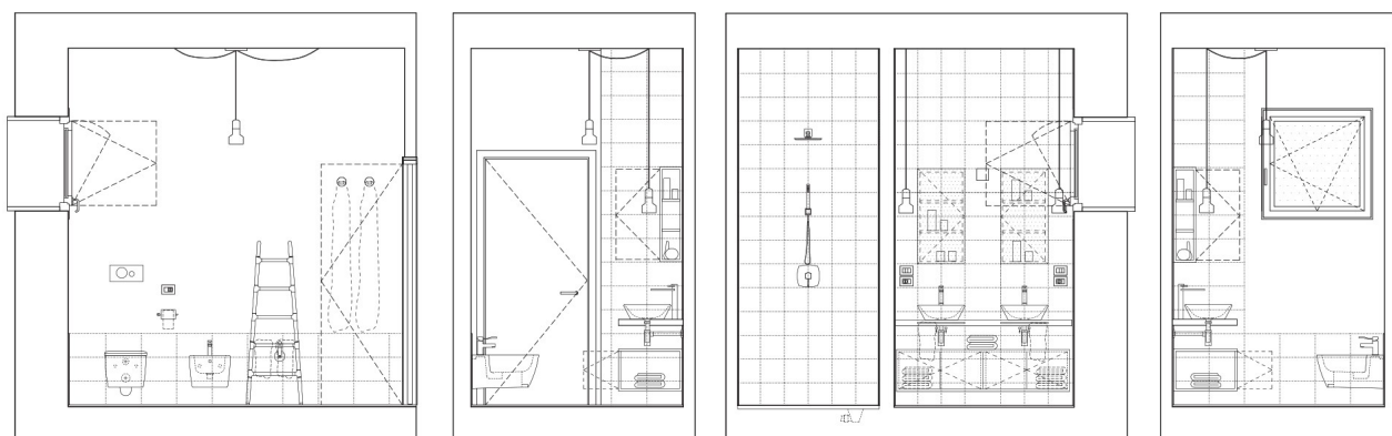
LATO A
